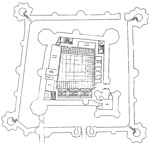
PLANTA BAJA
