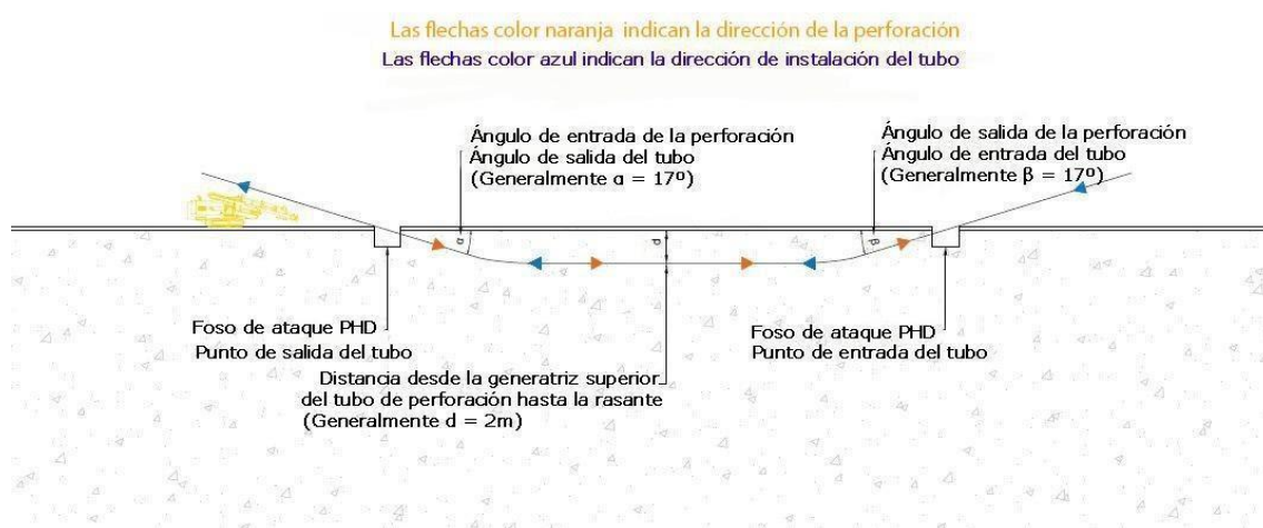
Figura 6. Esquema de perforación e instalación del tubo cruzamiento en la carretera CL-607
